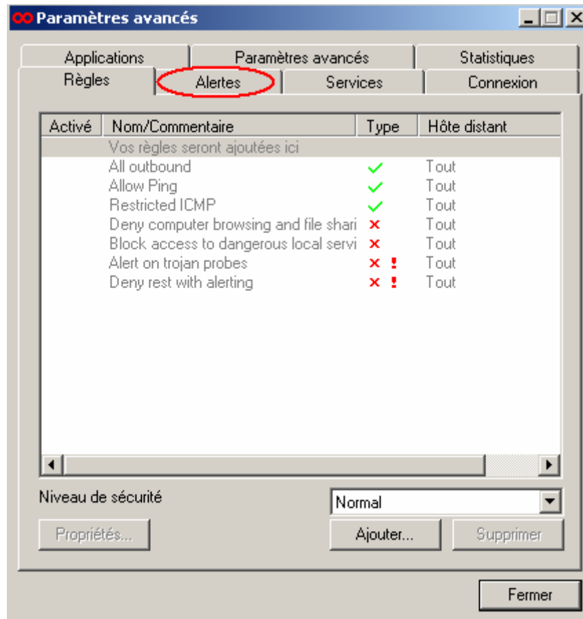
Figure 3 : Fenêtre des paramètres avancés du Firewall
