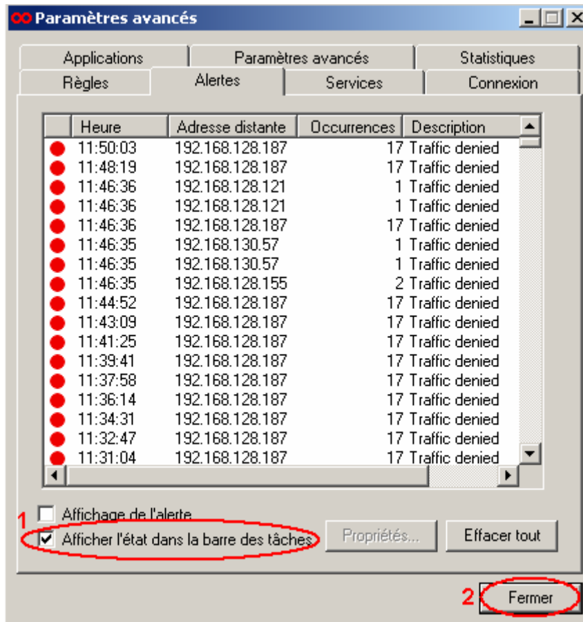
Figure 4 : Fenêtre des options de l'onglet alertes
