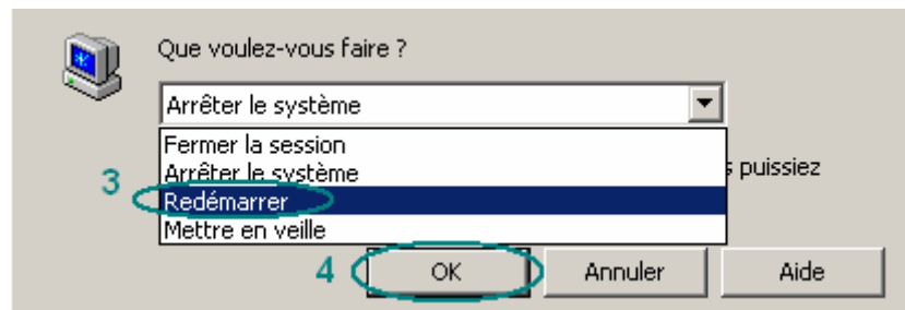
Figure 5 : Redémarrer l'ordinateur
