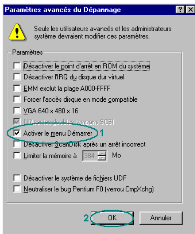
Figure 7 : Fenêtre "Paramètres avancés du dépannage"
