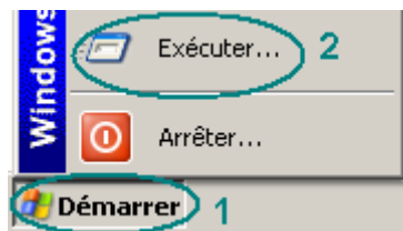
Figure 12 : Menu Démarrer
