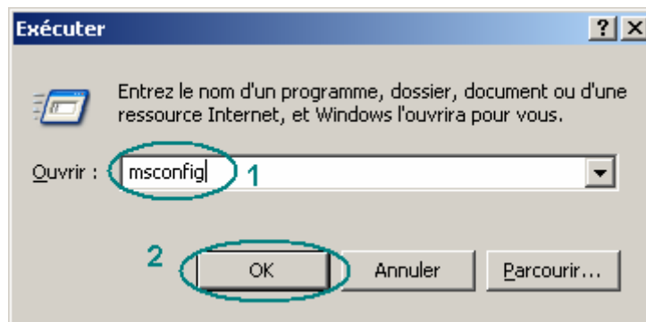
Figure 19 : Exécuter
