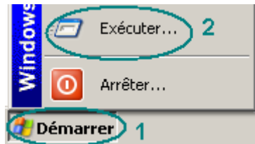
Figure 22 : Exécuter
