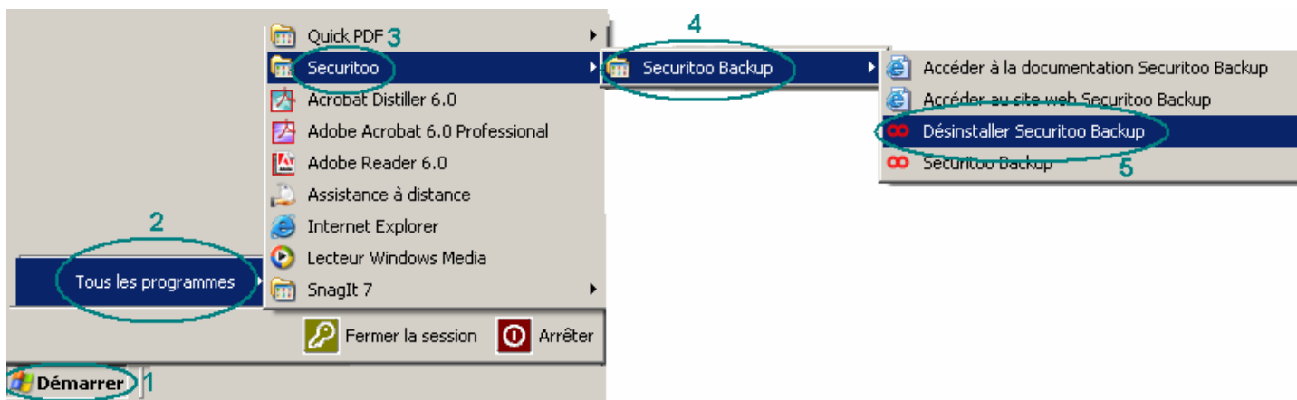
Figure 1 : Désinstaller Backup
