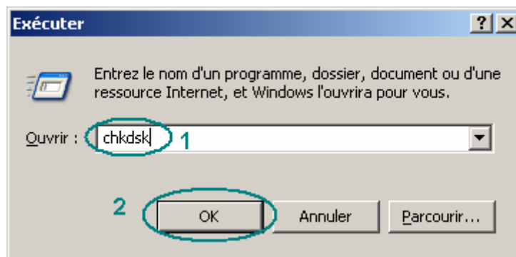
Figure 4 : « chkdsk »
