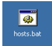
Figure 4 : Fichier « hosts.bat »
