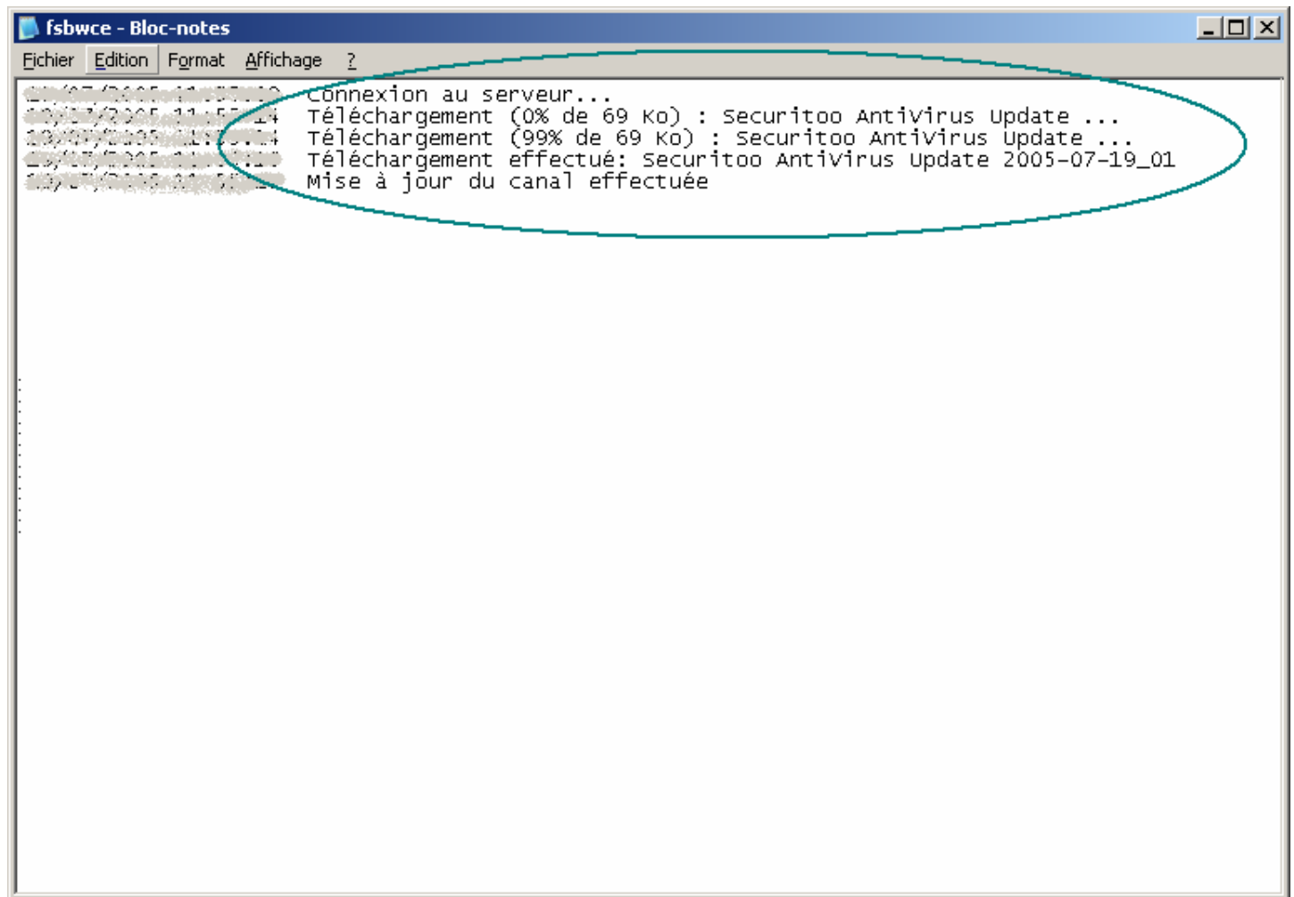
Figure 10 : Fichier journal
