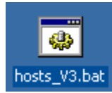
Figure 4 : Fichier « hosts_V3.bat »
