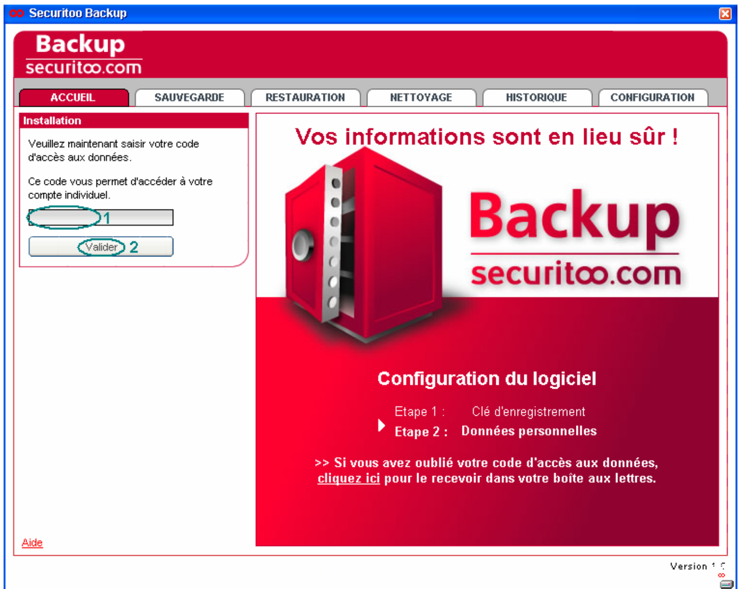
Figure 10 : Code d'accès
