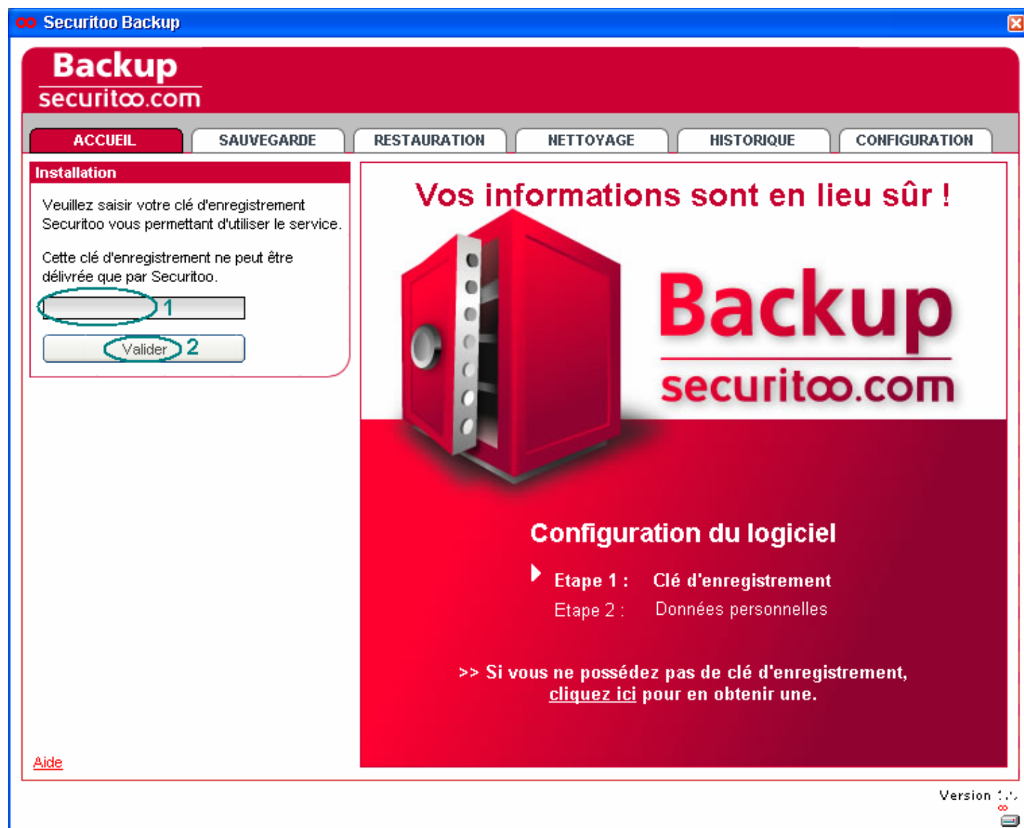
Figure 9 : Clé d'enregistrement
