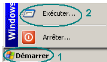
Figure 7 : Exécuter
