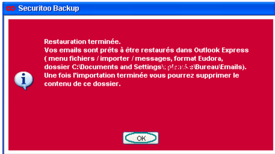
Figure 6 : Restauration terminée
