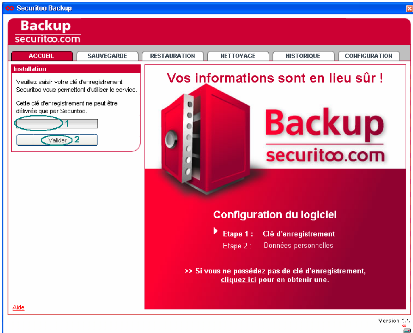
Figure 2 : Clé d'enregistrement
