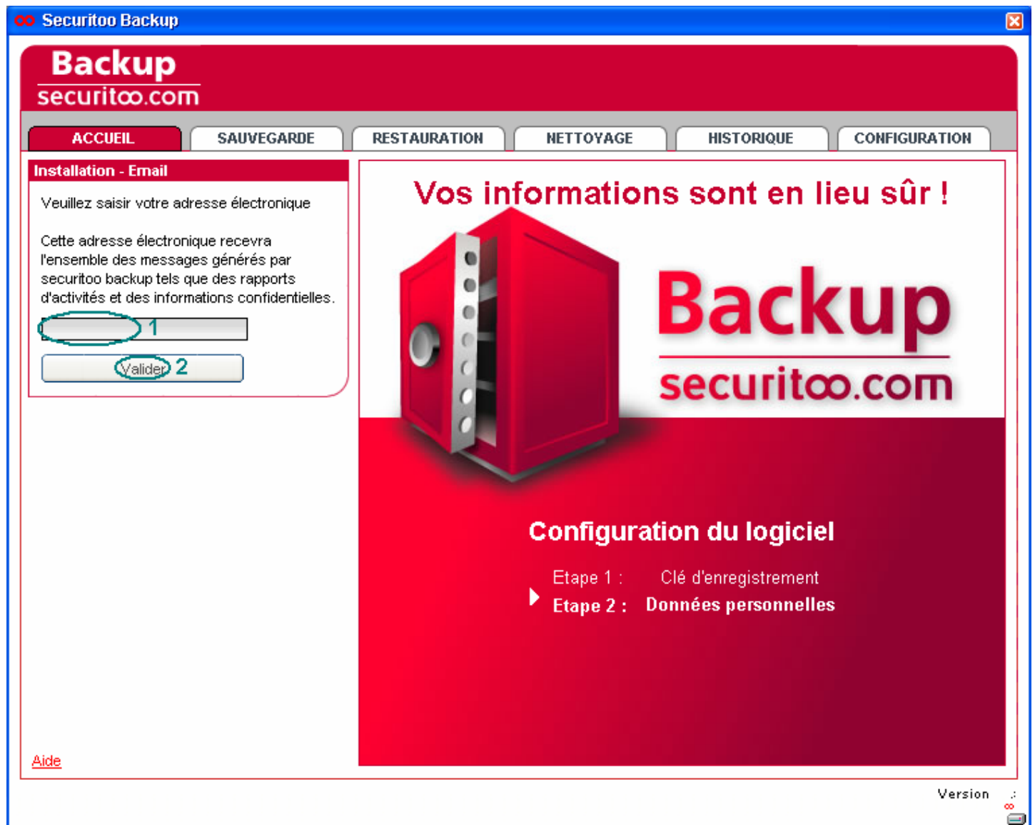
Figure 4 : Adresse email
