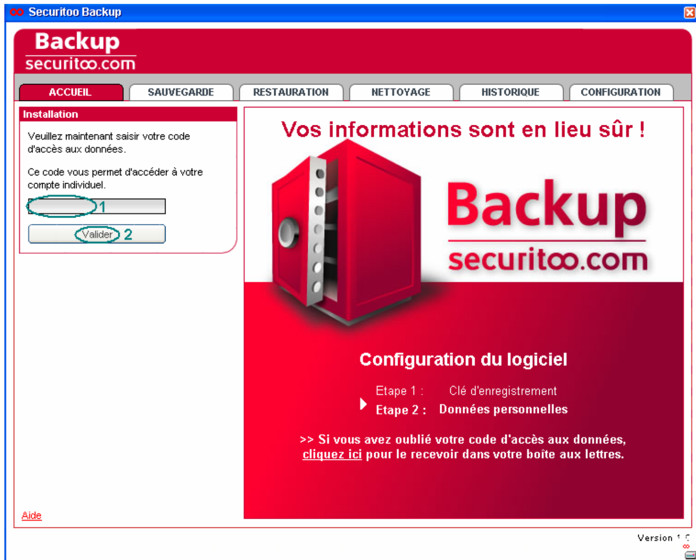
Figure 3 : Code d'accès
